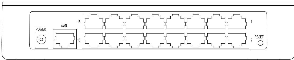
图2-2 TL-R1660+后面板示意图
